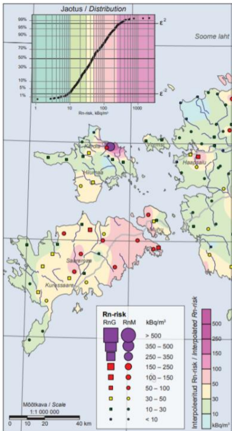
Joonis 22. Maksimaalne 222 Rn-sisaldus pinnaseõhus (kBq/m 3 ). Allikas: Eesti pinnase radooniriski ja looduskiirguse atlas. Eesti Geoloogiakeskus, Tallinn 2017 (väljavõte kaardist 6.1)
