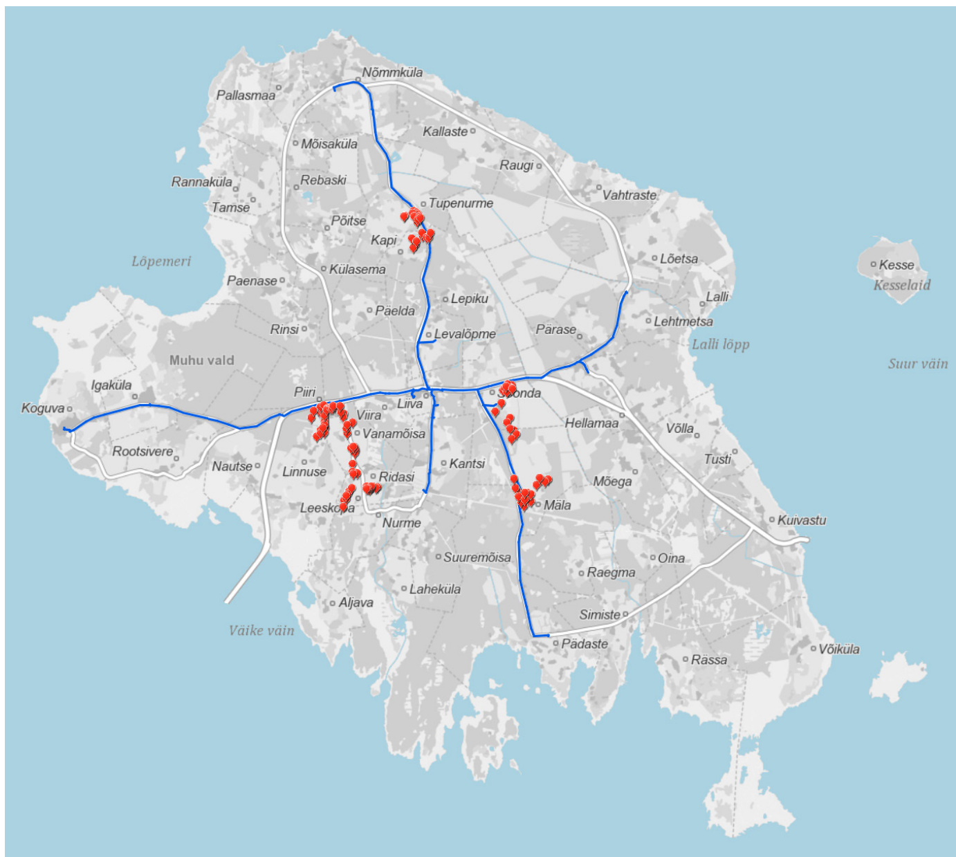
Joonis 17. 2024. a jaanuari seisuga ELA magistraalvõrk (sinisega ca 36 km) ja Enefit Connect ühendused (punasega ca 128 liitumispunkti) Allikas: Digisaar.ee
