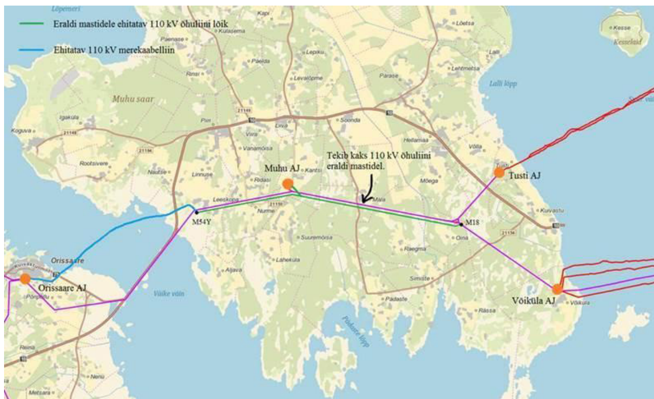
Joonis 16. 2022. a valminud täiendav õhuliin Muhus. Allikas: Elektrilevi
