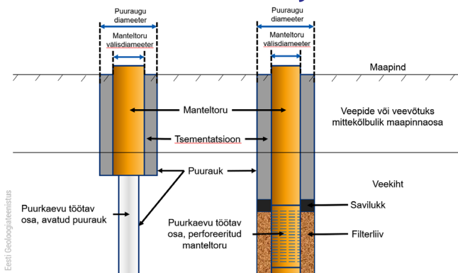
Joonis 1. Puurangu ja puurkaevu ehituslikud komponendid. Eestis kasutatakse puurkaevude rajamisel enamasti kolme meetodit: klassikaline puurkaevu rajamine, topeltpöördpeaga puurmasinaga puurkaevu rajamine ning puurkaevu rajamine ODEX tehnoloogial põhinevat puurimisviisi kasutades.
