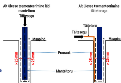
Joonis 2. Puurkaevu tsementeerimine peab toimuma alt ülesse meetodil kas läbi manteltoru või läbi spetsiaalse täitetoru, mis ulatub puurangu põhjani.
