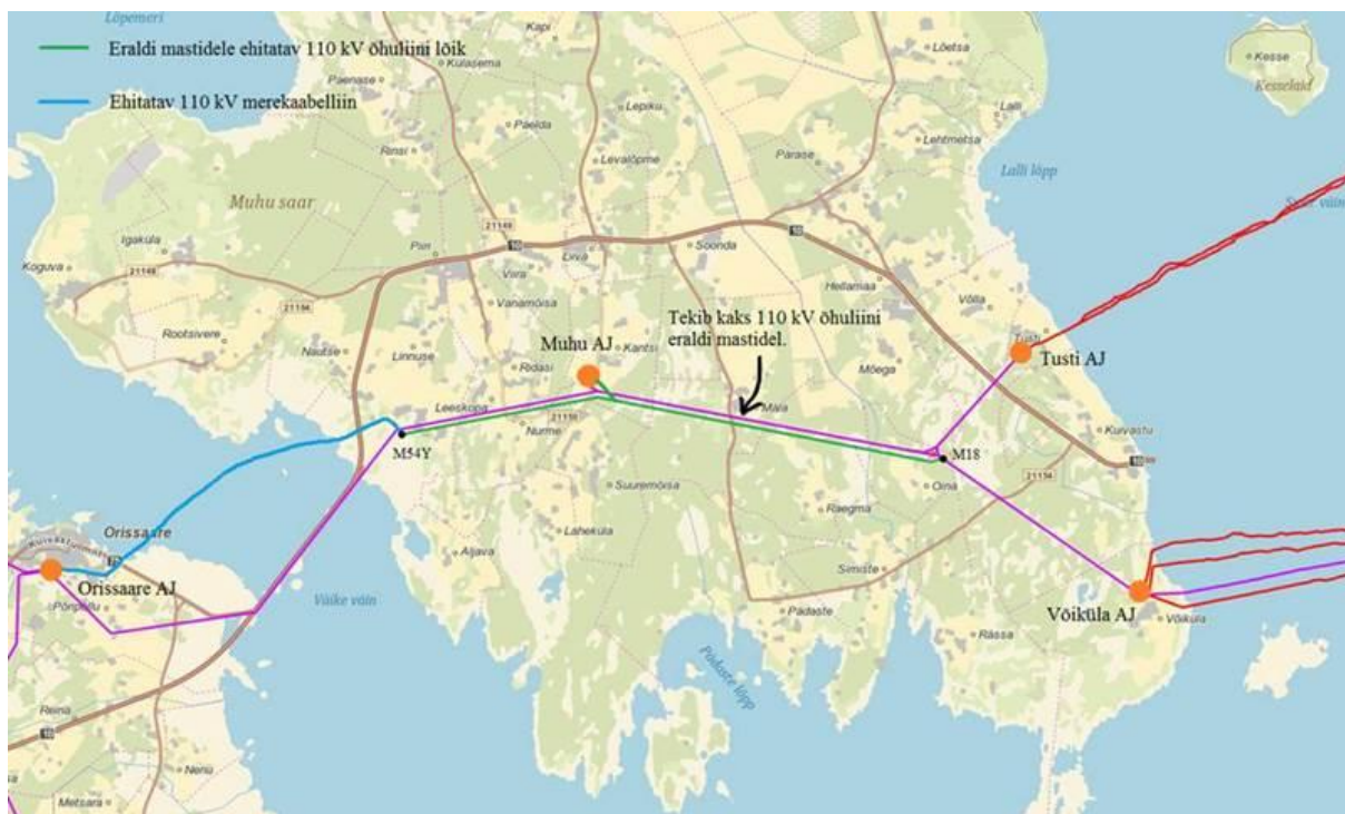
Joonis 9. Kavandatav täiendav õhuliin Muhus
