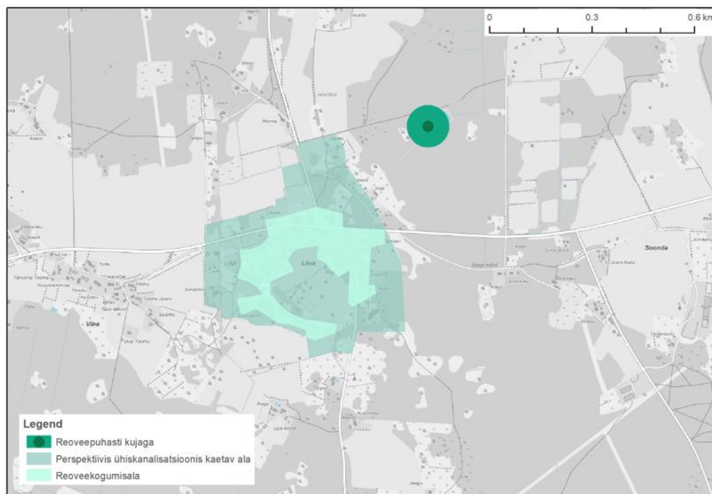
Skeem 6.10.1. Liiva küla reoveekogumisala 59 ja perspektiivis ühiskanalisatsiooniga kaetav ala.
